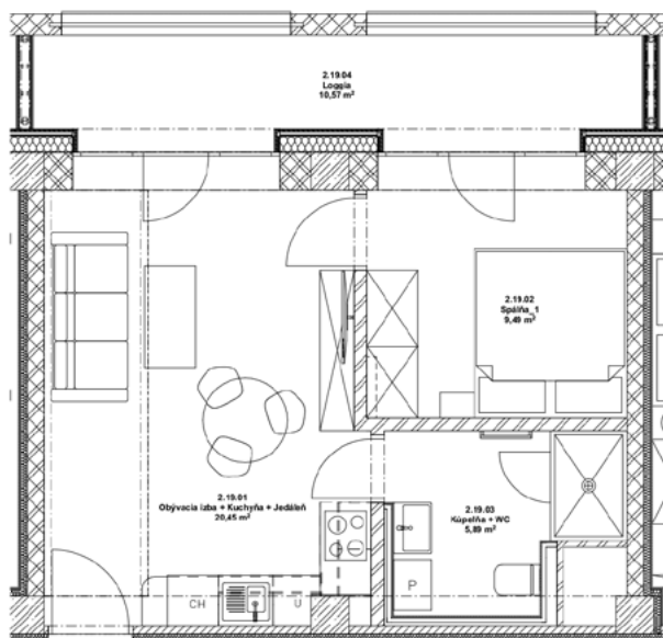
19.A Apartmán : 19.A 1:50
